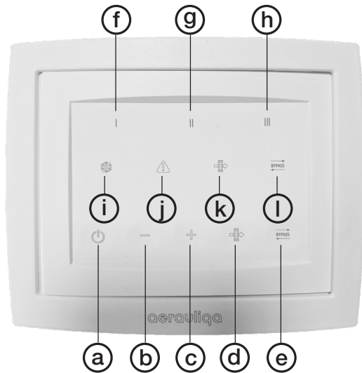
Fig. 7.a CTRL-V2
