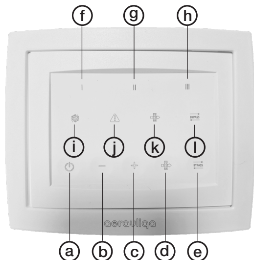
Fig. 7.a CTRL-V2
