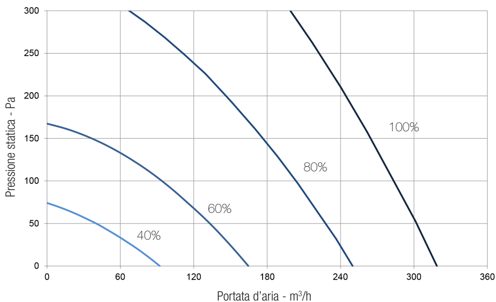
Fig. 6.b Curva di immissione in accordo al Reg. 1253/2014 (ErP).
