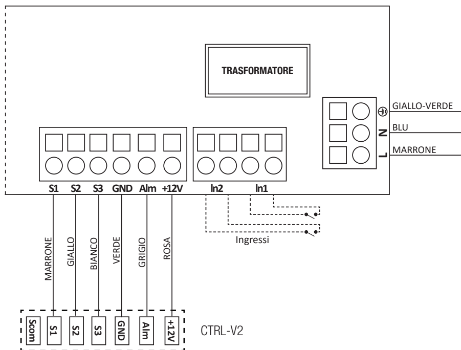
Fig. 5.m Collegamenti elettrici sulla scheda madre fissata all'interno della scatola collegamenti elettrici
