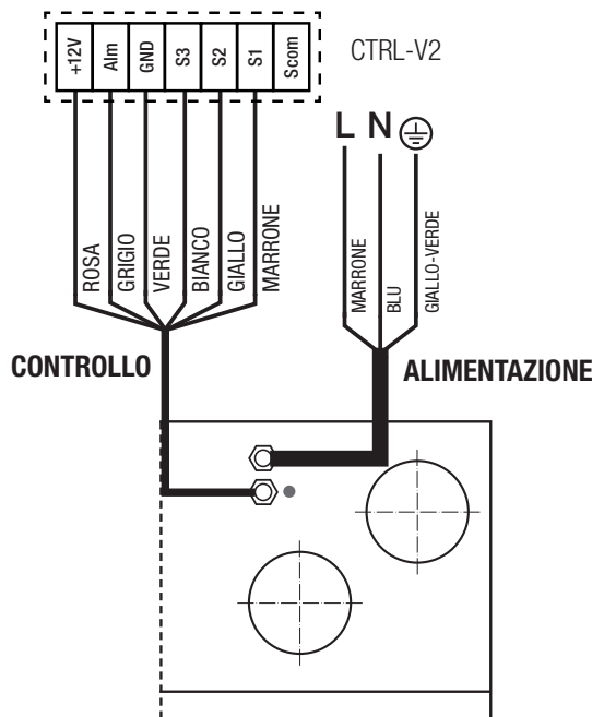
Fig. 5.k Precablaggio
