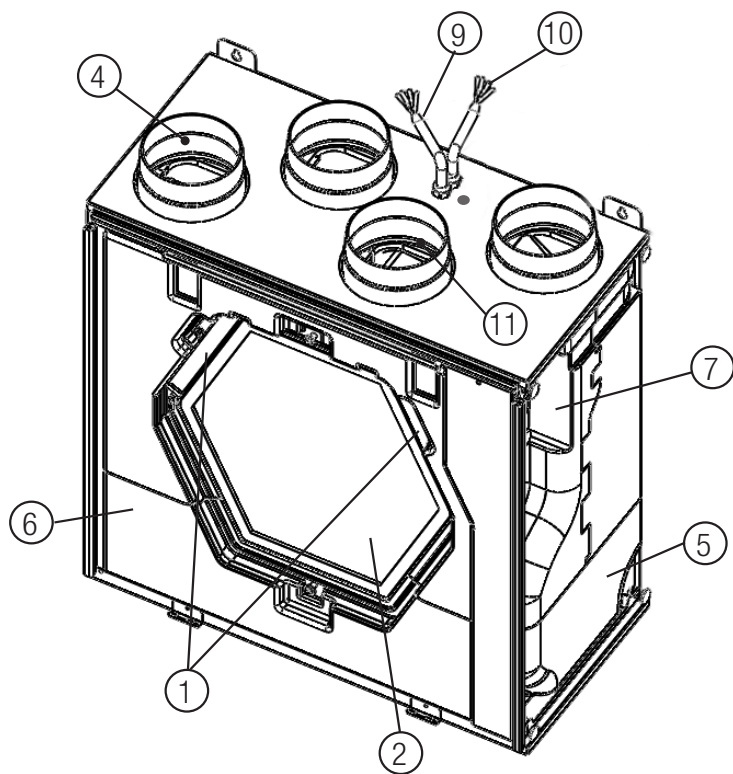
Fig. 8.a Componenti interni
