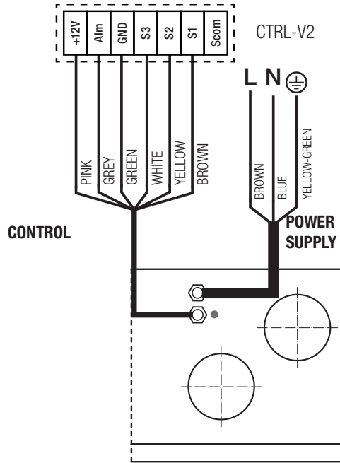
Fig. 5.k Precabing
