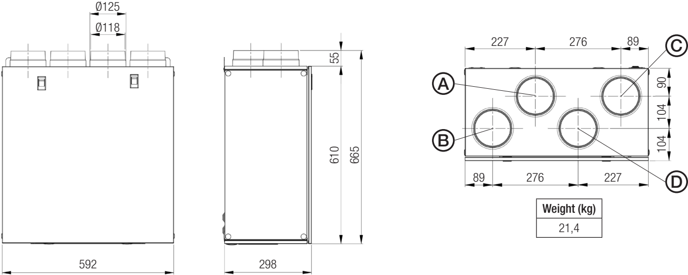
Fig. 3.a Dimensions (mm)
