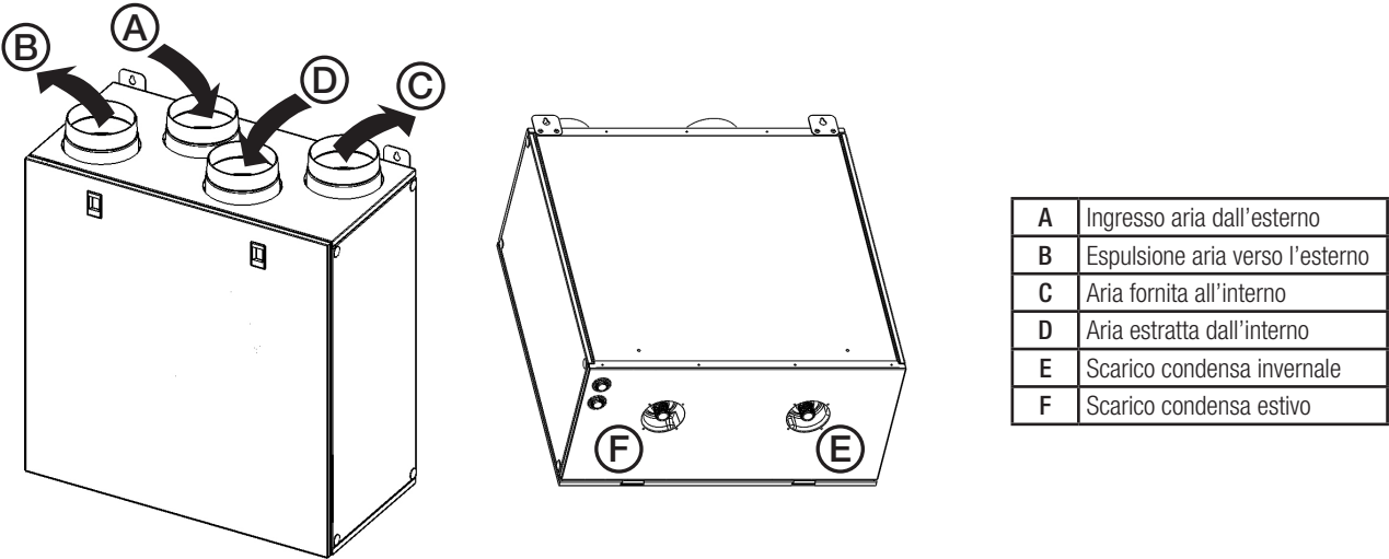
Fig. 3.b Connessioni
