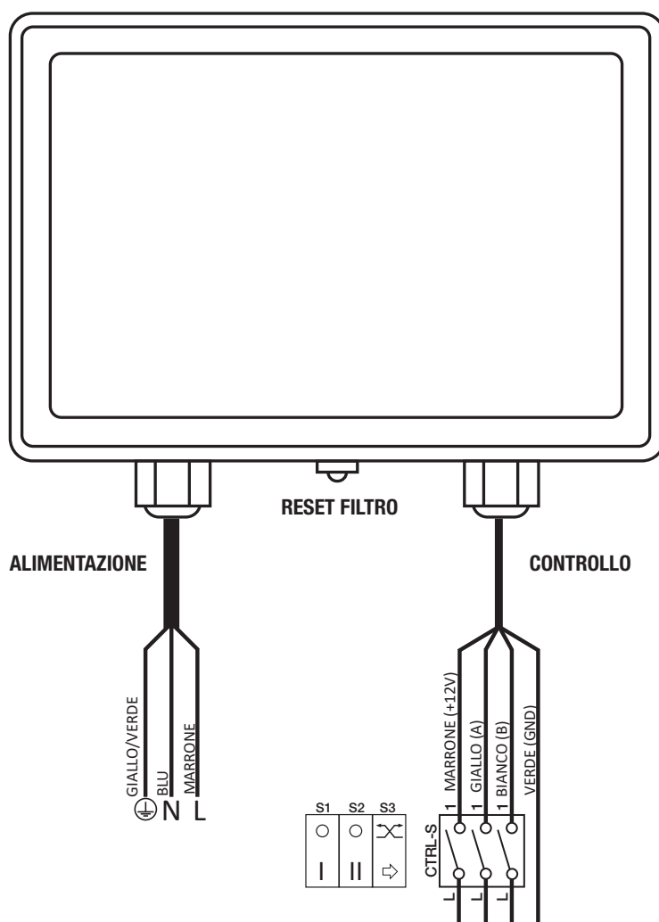
Fig. 5.f Collegamento cavi
