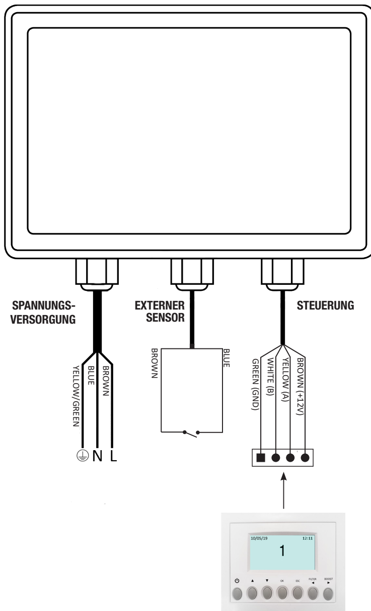
Abb. 5.f Elektronische Anschlüsse
