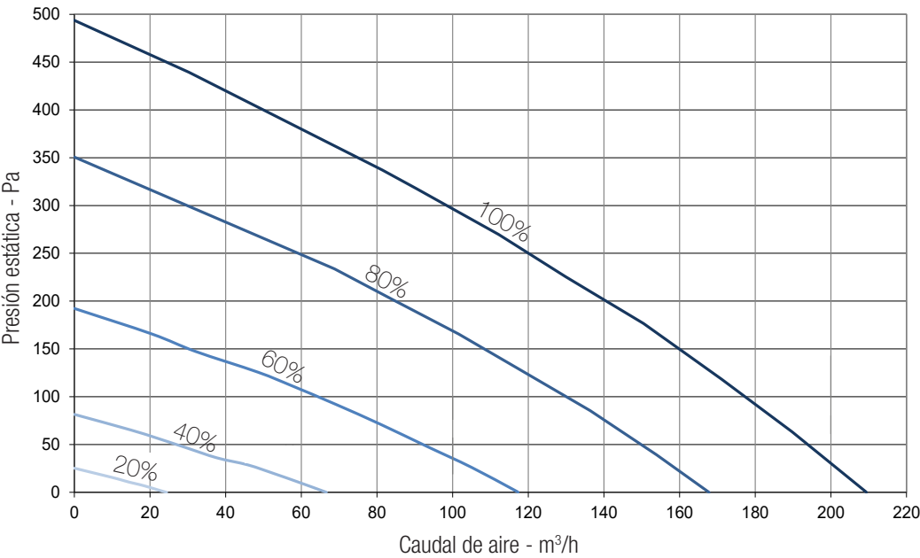
Fig. 6.a Curva de entrada según el Reg. 1253/2014 (ErP).
