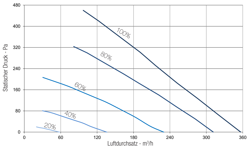
Abb. 6.d Zuluftkurven gemäss Reg. 1253/2014 (ErP)
