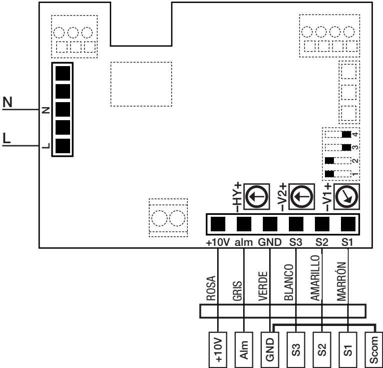
Fig. 5.q Conexiones eléctricas en la placa base de la máquina.
