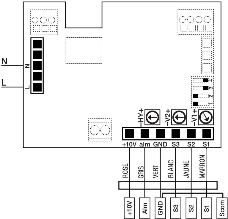
Fig. 5.q Connexions électriques au circuit de l'unité.
