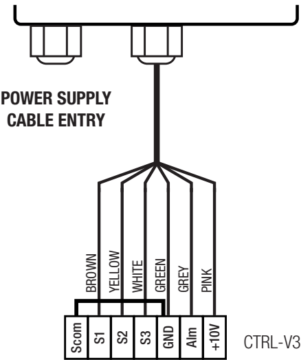
Fig. 5.o Precabling
