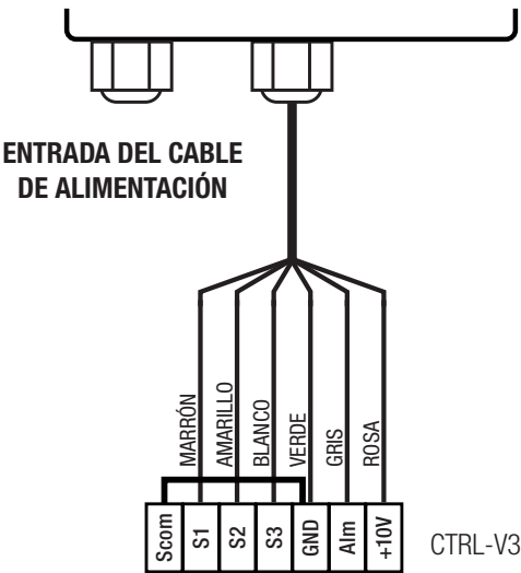
Fig. 5.o Precableado del mando
