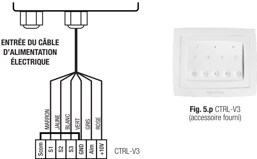
Fig. 5.o Précâblage du contrôleur
