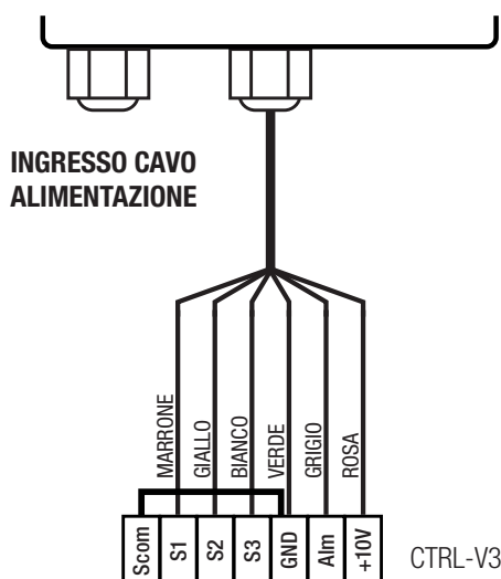
Fig. 5.o Precablaggio comando
