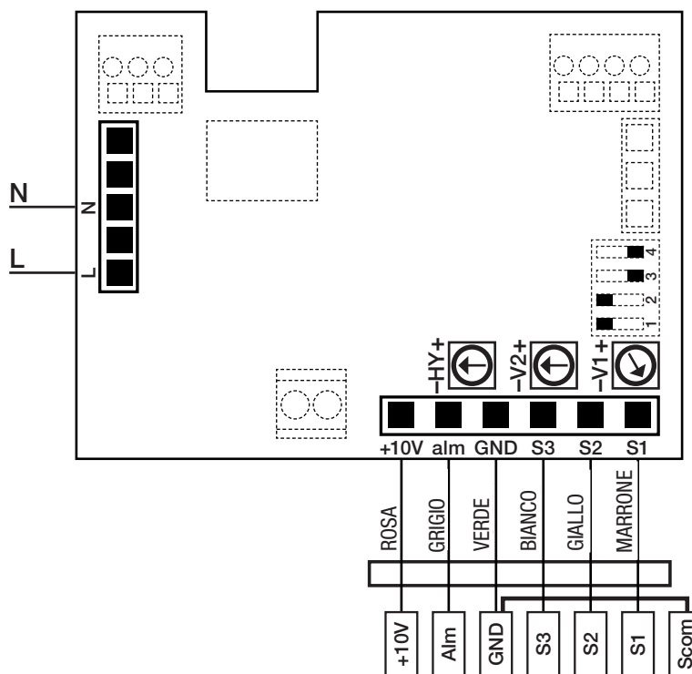
Fig. 5.q Collegamenti elettrici sulla scheda madre a bordo macchina.
